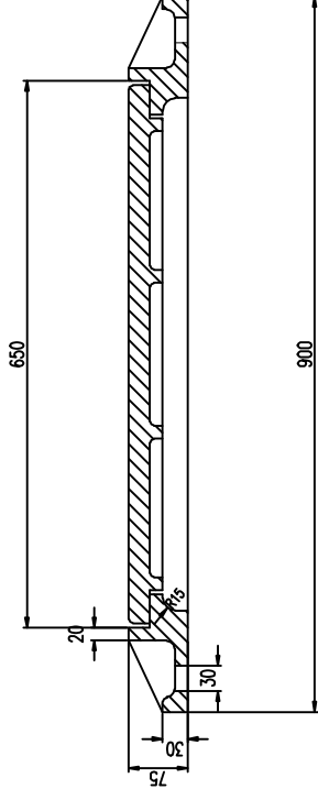
Mặt cắt a-a Section a-a
